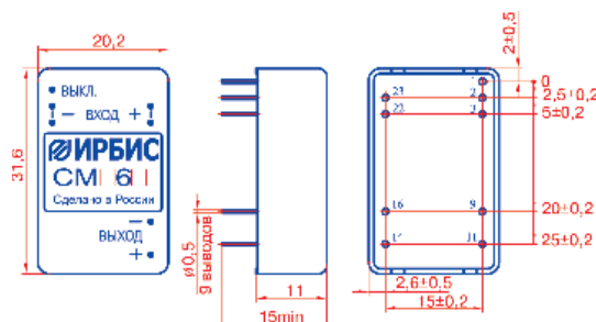
Номера выводов показаны условно
